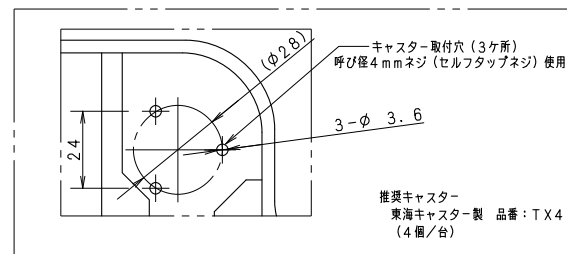
キャスター取付用 参考寸法図
